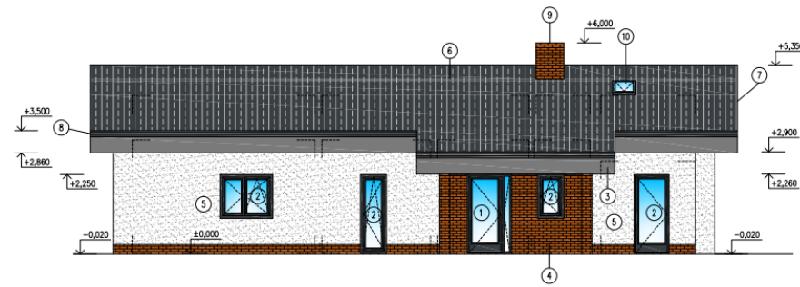
BOČNÍ PRAVÝ POHLED
