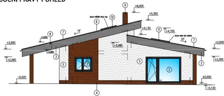
BOČNÍ PRAVÝ POHLED
