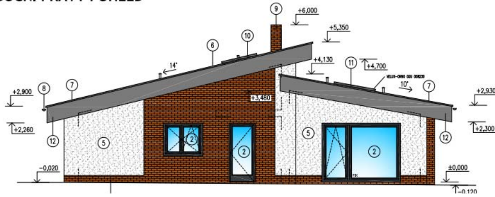
BOČNÍ PRAVÝ POHLED
