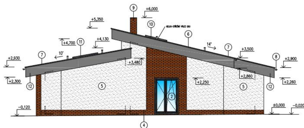
BOČNÍ LEVÝ POHLED
