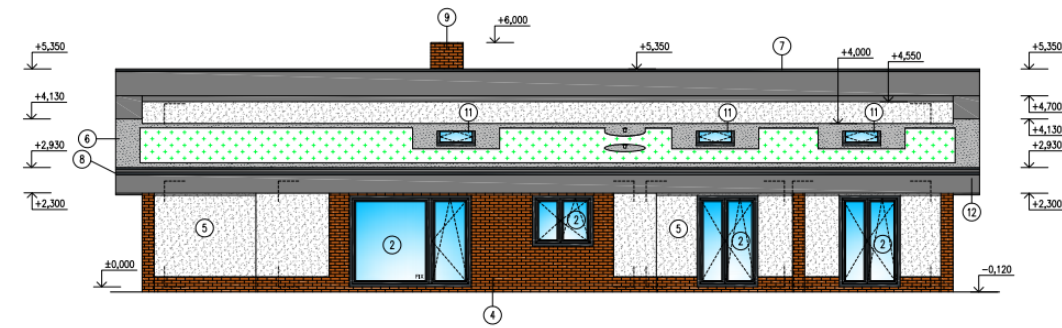
BOČNÍ LEVÝ POHLED
